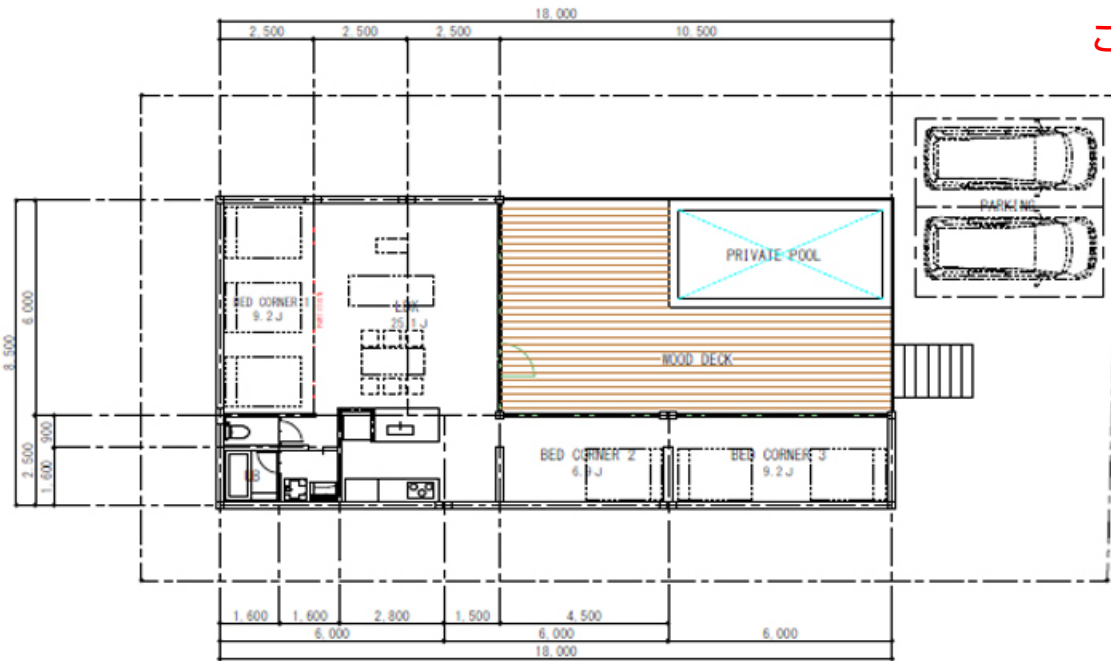
PLAN 1/150
