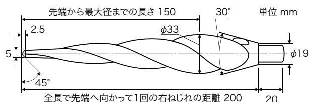
図1 スクリューポイント
